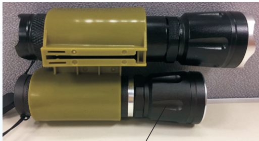
白光手电调焦：来回拉动前端灯头
